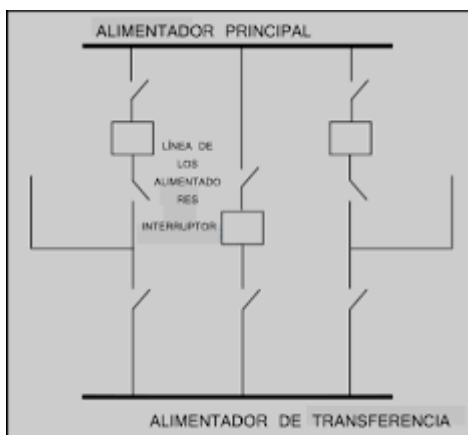
Figura 5-36 Bucle primario de distribución.
