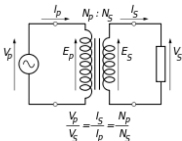
Figura 4-5 Relación de vueltas del transformador.
