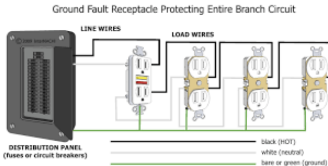
Figura 6-19 Circuito GFCI
