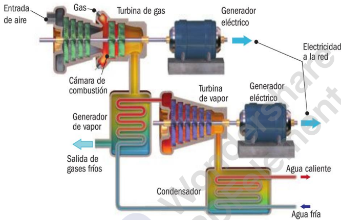
Figura 2-10 Planta de energía de ciclo combinado.
