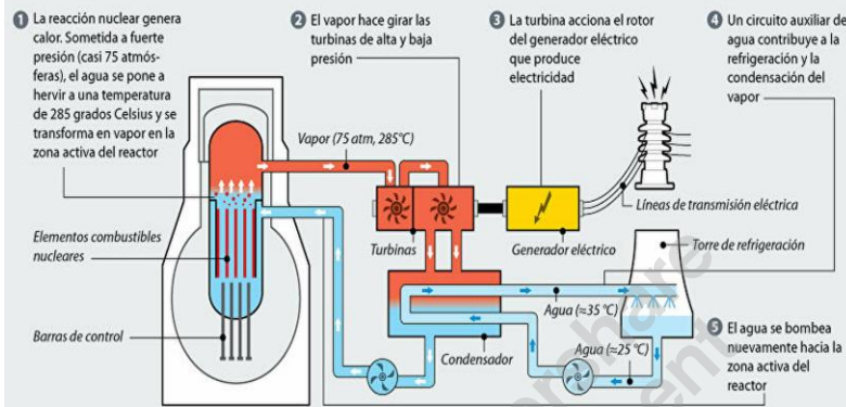
Figura 2-5 Reactor de agua en ebullición.
