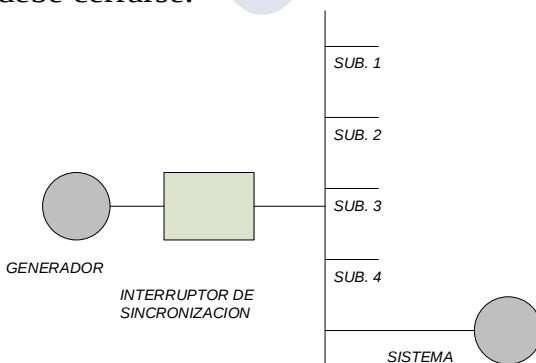
Figura 7-7 Sincronización del generador.
