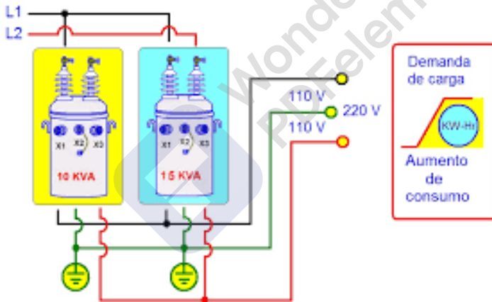
Figura 5-15 Conexiones de transformador de dos Bushing.
