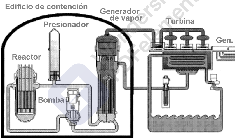
Figura 2-4 Reactor de agua a presión.
