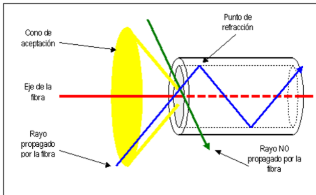
Figura 9-8 Principios de fibra óptica.
