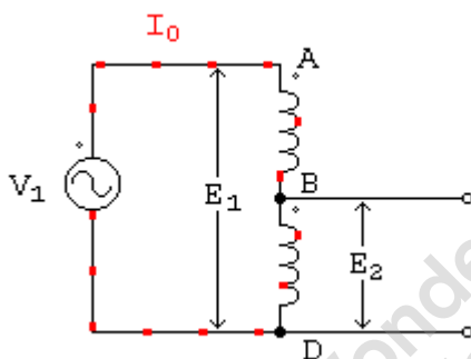
Figura 4-16 Autotransformador.
