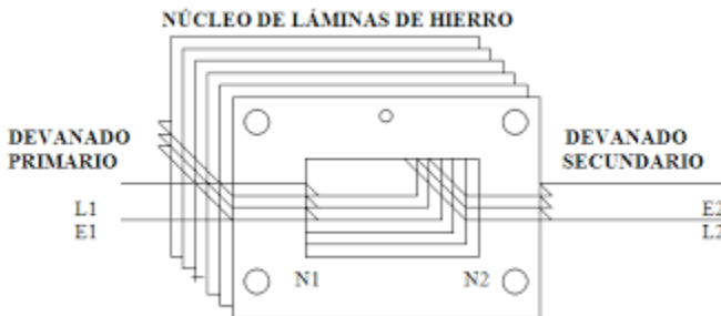
Figura 4-4 Devanados del transformador.
