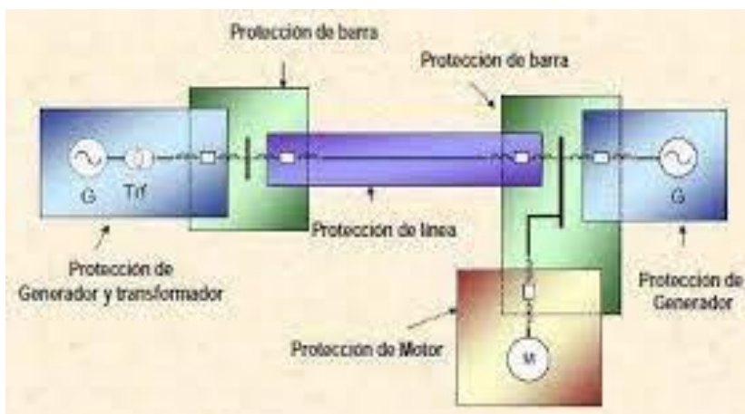
Figura 7-9 Protección de transmisión.
