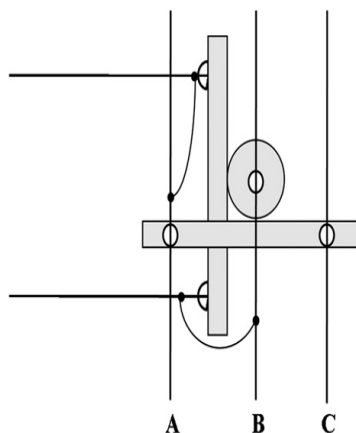
Figura 5-11 Lateral Delta monofásico. Cortesía de Alliant Energy.
