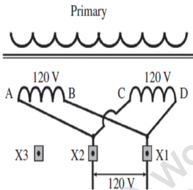
Figura 5-20 Conexión # 2 del banco de transformadores.
