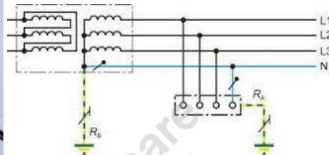
Figura 5-6 Alimentador trifásico en Wye Cortesía de Alliant Energy.
