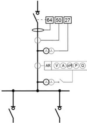
Figura 7-4 Diagrama unifilar.
