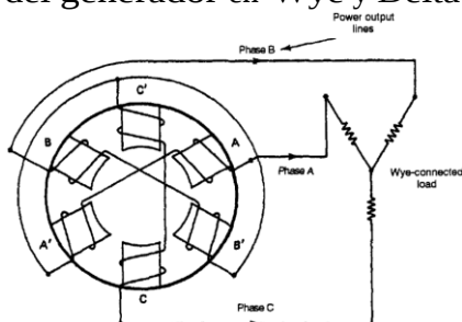
Figura 1-14 Generador conectado en Wye.
