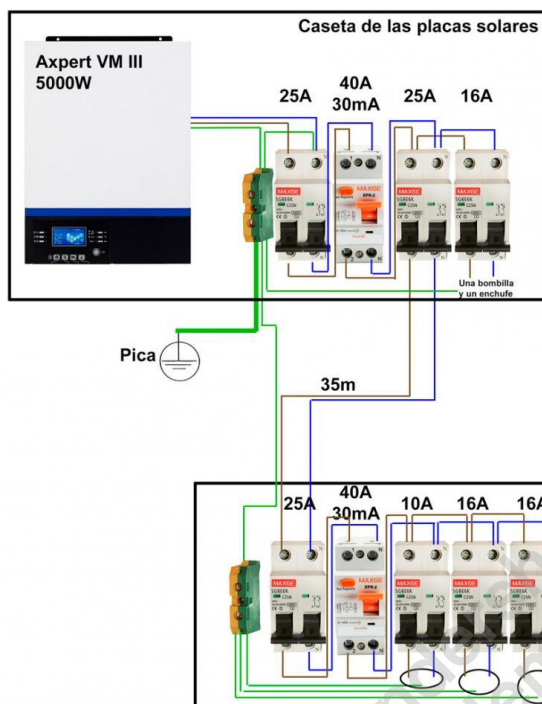
Figura 6-16 Cuadro eléctrico – residencial.
