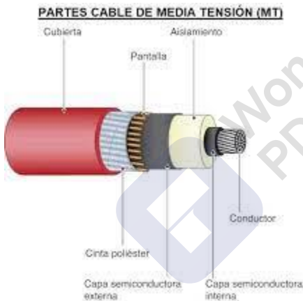
Figura 5-28 Cable de distribución principal de un solo conductor.
