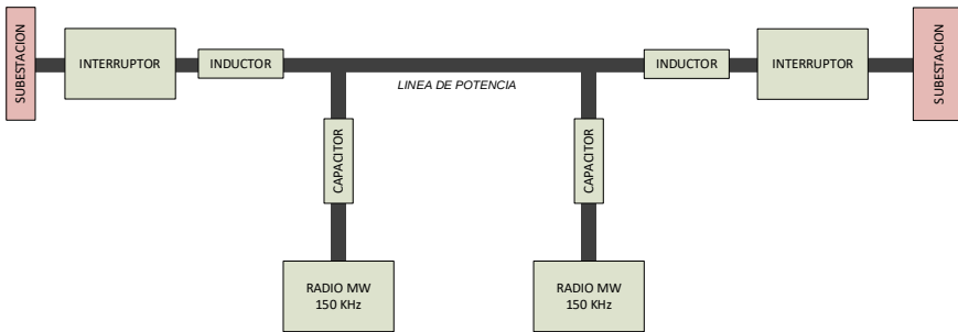
Figura 9-13 Portador de línea eléctrica.
