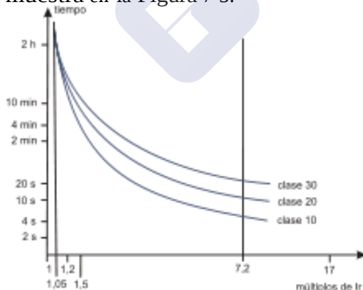
Figura 7-3 Curva Tiempo vs. Corriente
