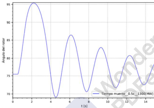
Figura 8-8 Sistema estable.
