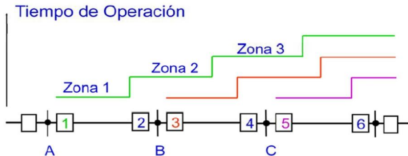
Figura 7-6 Protección de zona.
