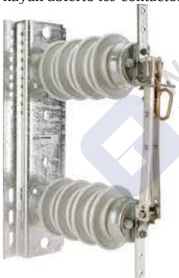
Figura 4-36 Varillas de arco.
