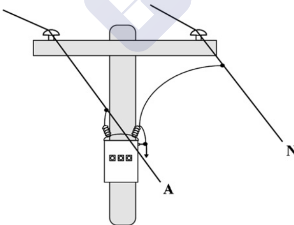
Figura 5-8 Lateral monofásico. Cortesía de Alliant Energy.
