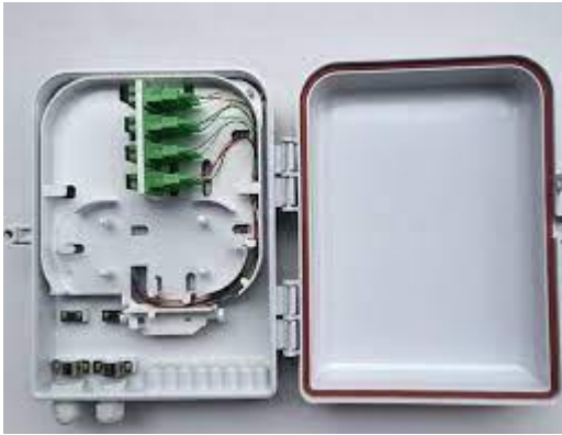
Figura 9-10 Terminación de fibra.
