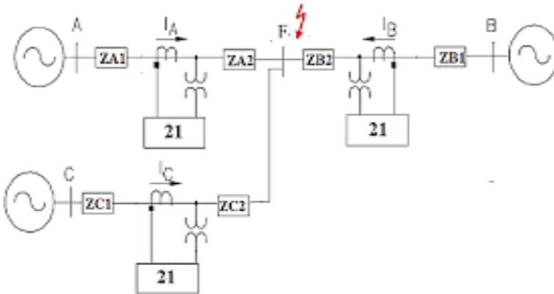
Figura 7-5 Falla en el sistema de transmisión.
