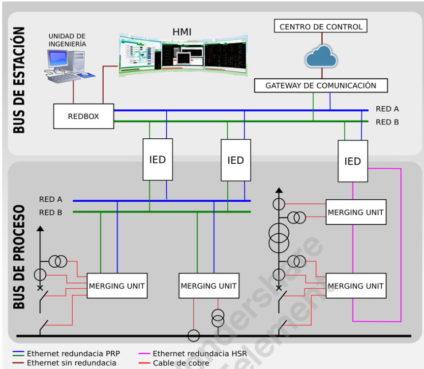
Figura 7-11 Subestación digital.
