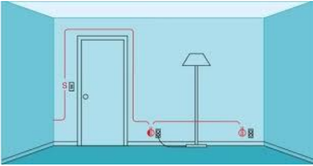
Figura 6-18 Circuito del receptáculo.
