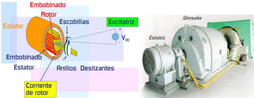
Figura 1-12 Excitatriz
