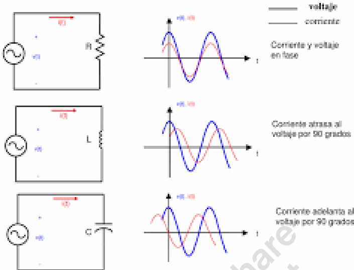
Figura 6-2 Relaciones de tensión y corriente.
