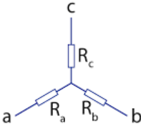
Figura 5-3 Conexión Estrella .
