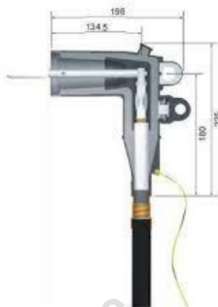
Figura 5-31 Ruptura de Carga de carga.
