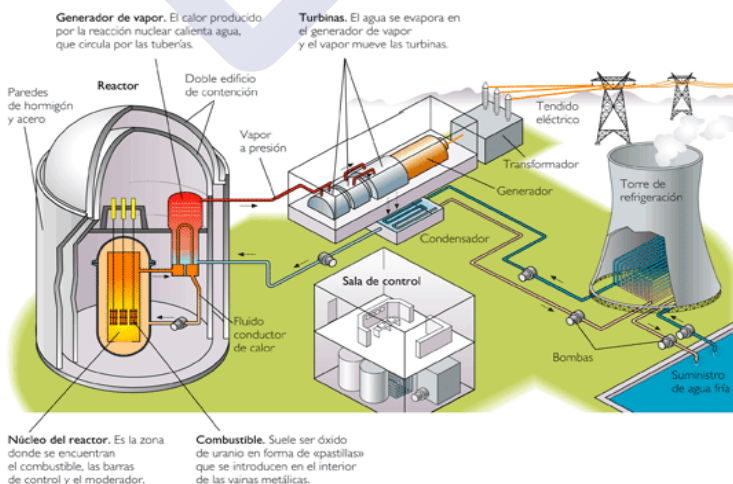
Figura 2-3 Planta de energía nuclear.
