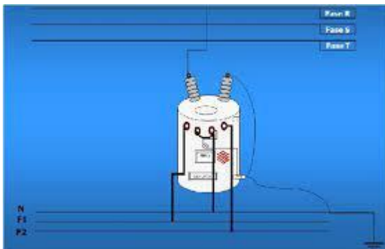
Figura 5-13 Conexiones del transformador.
