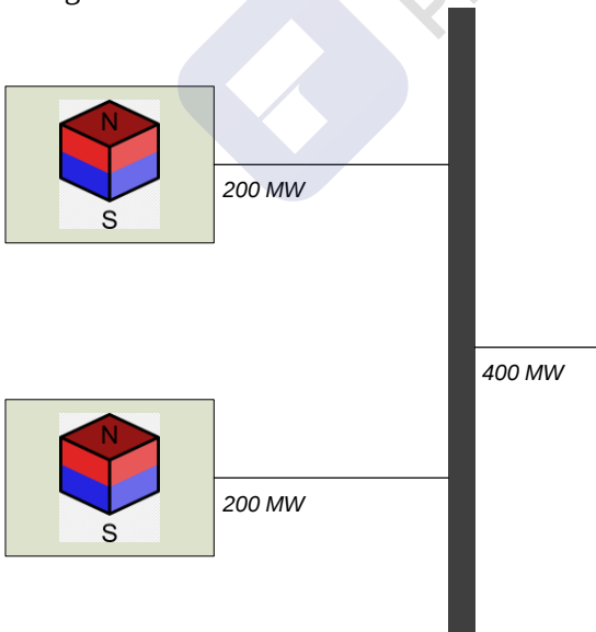
Figura 8-6 Generación equilibrada.
